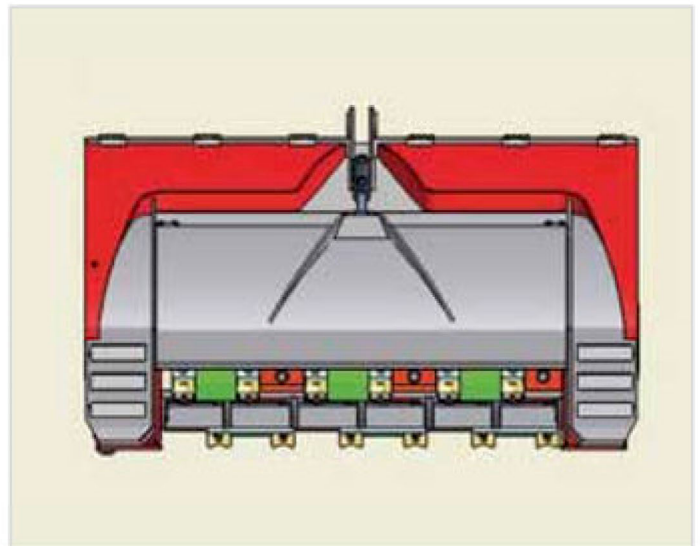
FRONTANSICHT CRUSHER
