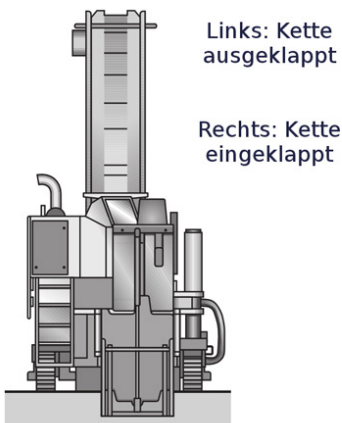
Prinzipische der Arbeitsweise von Kleinfräsen: Fräsrolle hinten rechts und Höhensteuerung über die Fahrwerke.
