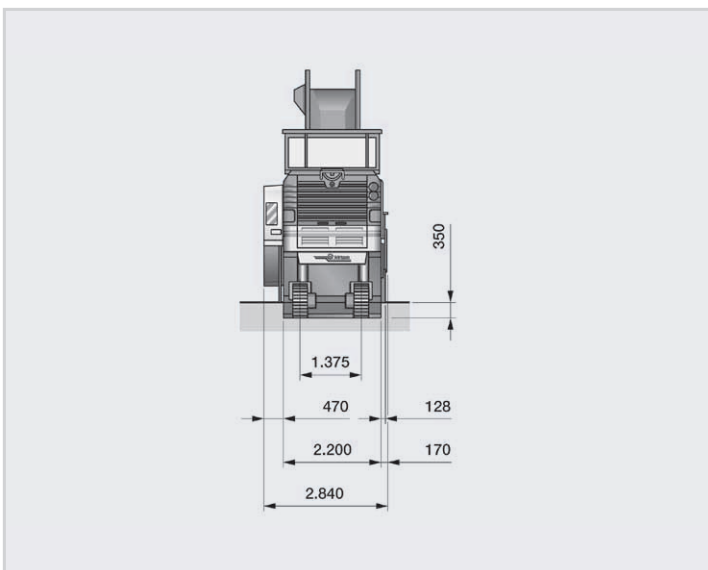
HECKANSICHT
